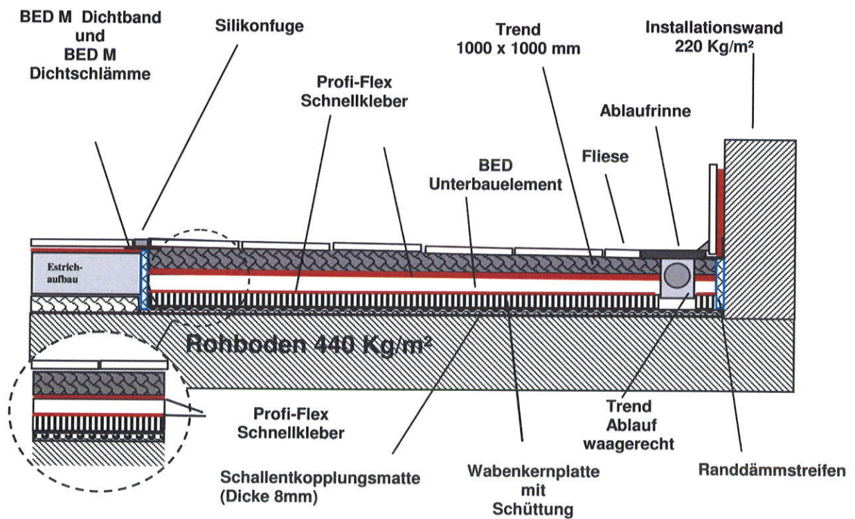
Bild 3 Lage des Duschsystems im Installationsraum EG vorne (oben) und Schnittzeichnung des Versuchsaufbaus mit Estrichanschluss (unten, Zeichnung des Auftraggebers).
